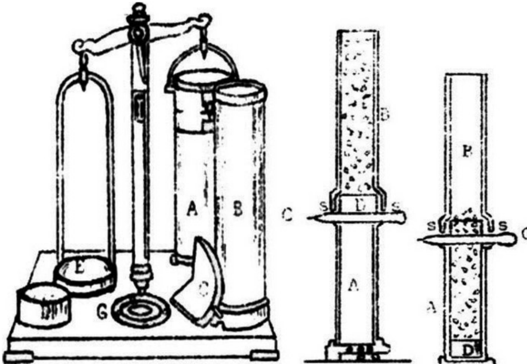
Figura 2: Equipo Schopper
